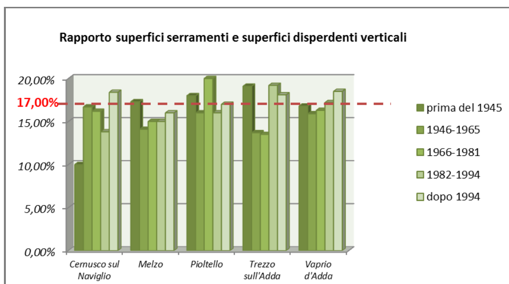
Grafico 3: Rapporto tra le superfici dei serramenti e le superfici disperdenti verticali
